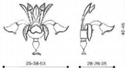
ALBINONI.A L.25 SP.28 H.40 1 FIAMMA xE14 40W L.38 SP.26 H.40 2 FIAMME xE14 40W L.53 SP.35 H.45 3 FIAMME xE14 40W
