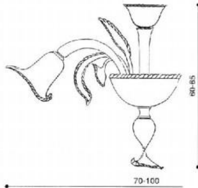
ALBINONI.R Ø 70 H.60 6 FIAMME xE14 40W Ø100 H.65 8 FIAMME xE14 40W
