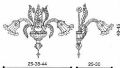
VIVALDI.A L.25 SP.25 H.40 1 FIAMMA xE14 40W L.38 SP.25 H.40 2 FIAMME xE14 40W L.44 SP.30 H.45 3 FIAMME xE14 40W
